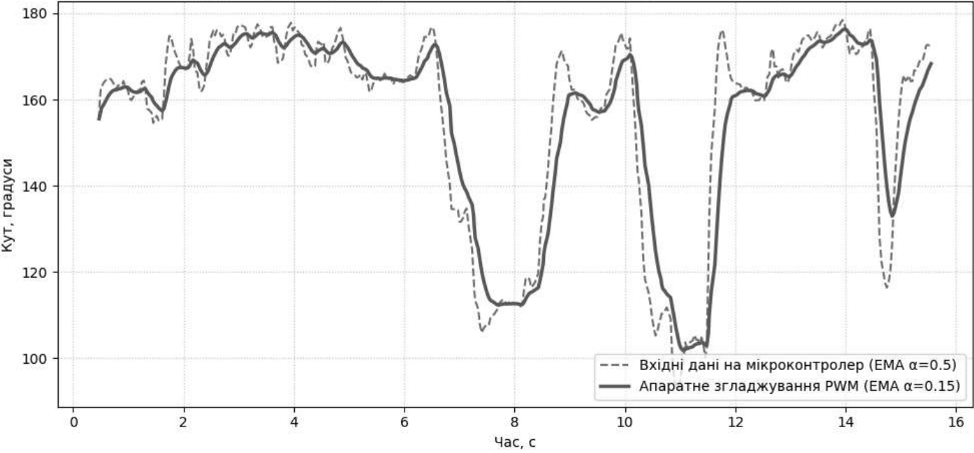
Другий рівень фільтрації: плавний рух сервопривода та поява затримки
