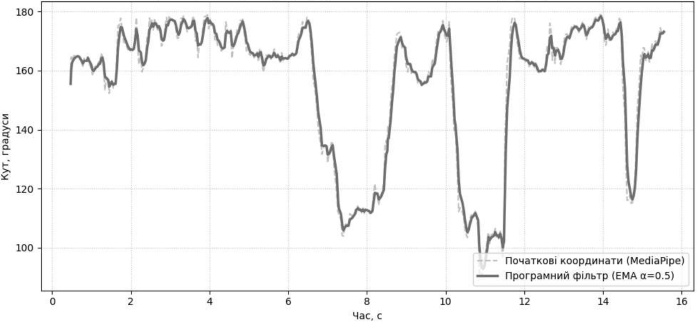
Перший рівень фільтрації: усунення високочастотного шуму на рівні ПК
